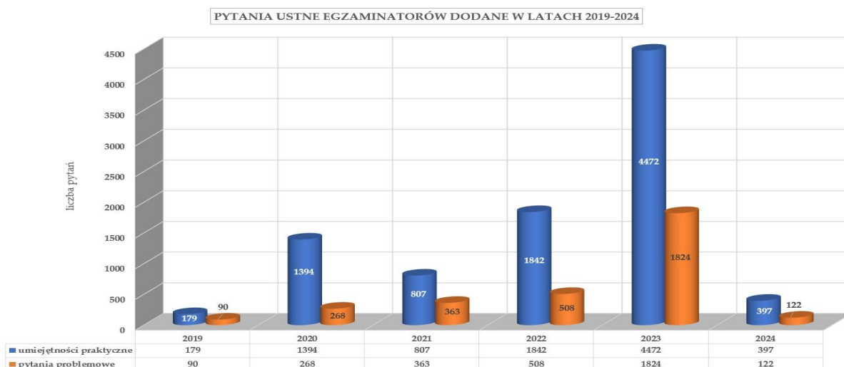
Rys. 5.1.1. Liczba wprowadzonych pytań ustnych do systemu SESZAT w latach 2019-2024.
