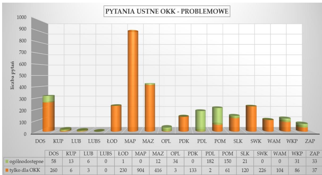
Rys. 5.1.6. Liczba pytań ustnych z grupy pytania problemowe z podziałem na ogólnodostępne i tylko dla OKK.
