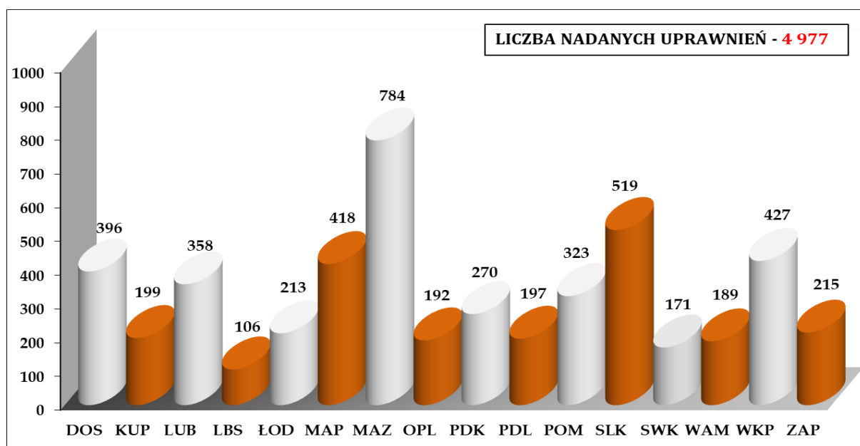
Rys. 5.2.2. Liczba osób, które uzyskały uprawnienia budowlane w 2024 roku w poszczególnych izbach okręgowych.
